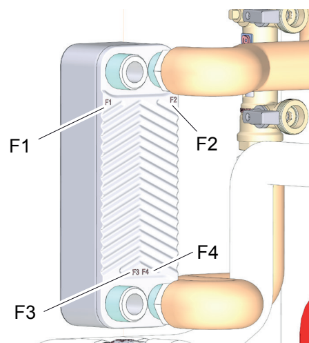
fig. 53 - dettaglio montaggio scambiatore a piastre
