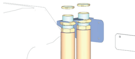
fig. 48 - dettaglio bloccaggio tubazioni su staffa superiore
