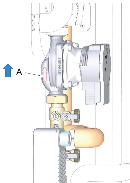
fig. 52 - dettaglio montaggio circolatore collettore solare
