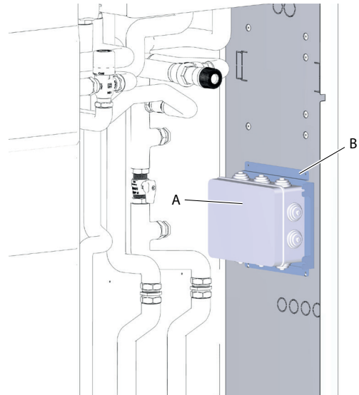
fig. 68 - scatola elettrica montata
