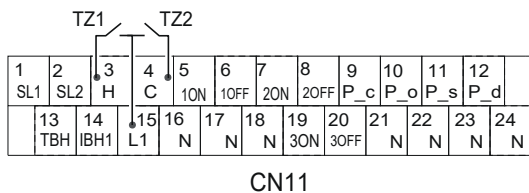
Morsettiere scheda idronica dell'unità interna
