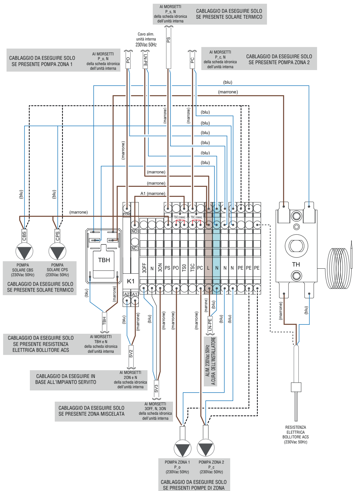
Morsettiere scheda idronica dell'unità interna
