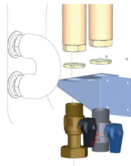
fig. 49 - dettaglio bloccaggio tubazioni su staffa inferiore
